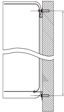
vertikale Montageposition
