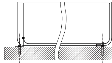
horizontale Montageposition
